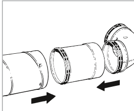
Liukuva naaras-liitoskappale
